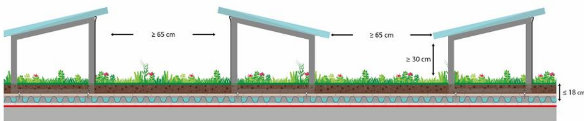
Bild 4 — Schematische Darstellung Solargründach mit Energiegewinnungselementen in Ost-Westausrichtung (im Schichtbau integriert) bis 18 cm
